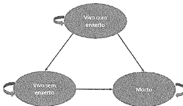
Figura 3 – Modelo de Markov apresentado pelo demandante.
