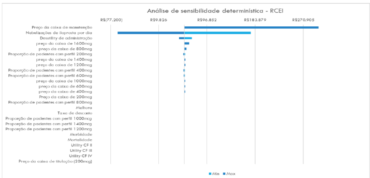
Figura 11: Gráfico de tornado da análise de sensibilidade determinística alternativa
