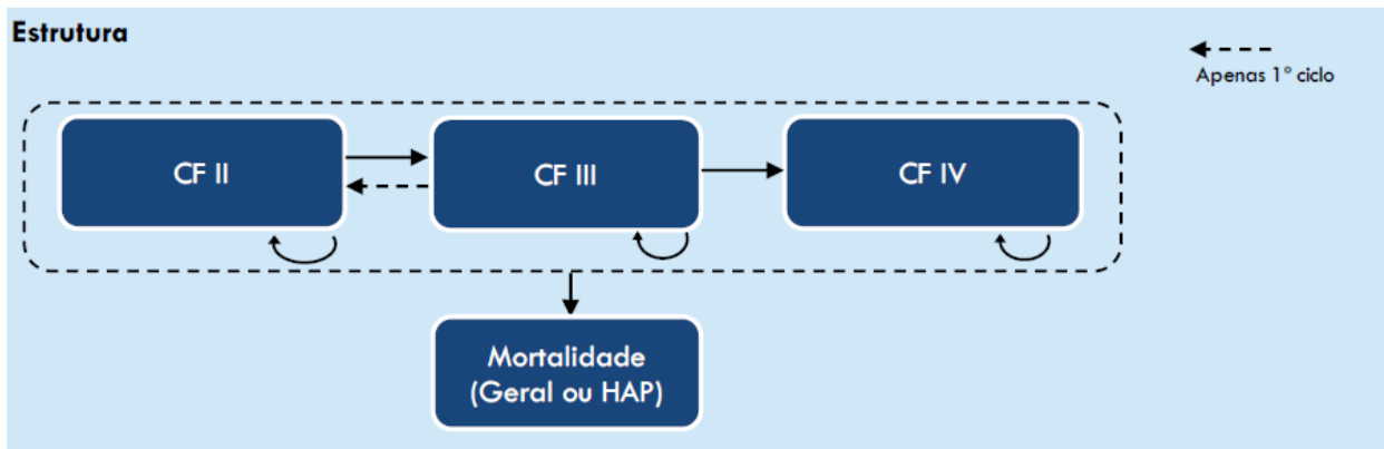
Figura 4: Estrutura do Modelo
