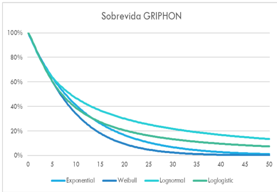
Figura 6: Curvas de sobrevivência – Estudo GRIPHON
