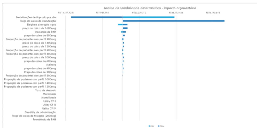
Figura 15: Análise de sensibilidade do cenário alternativo sem impostos – Gráfico de Tornado
