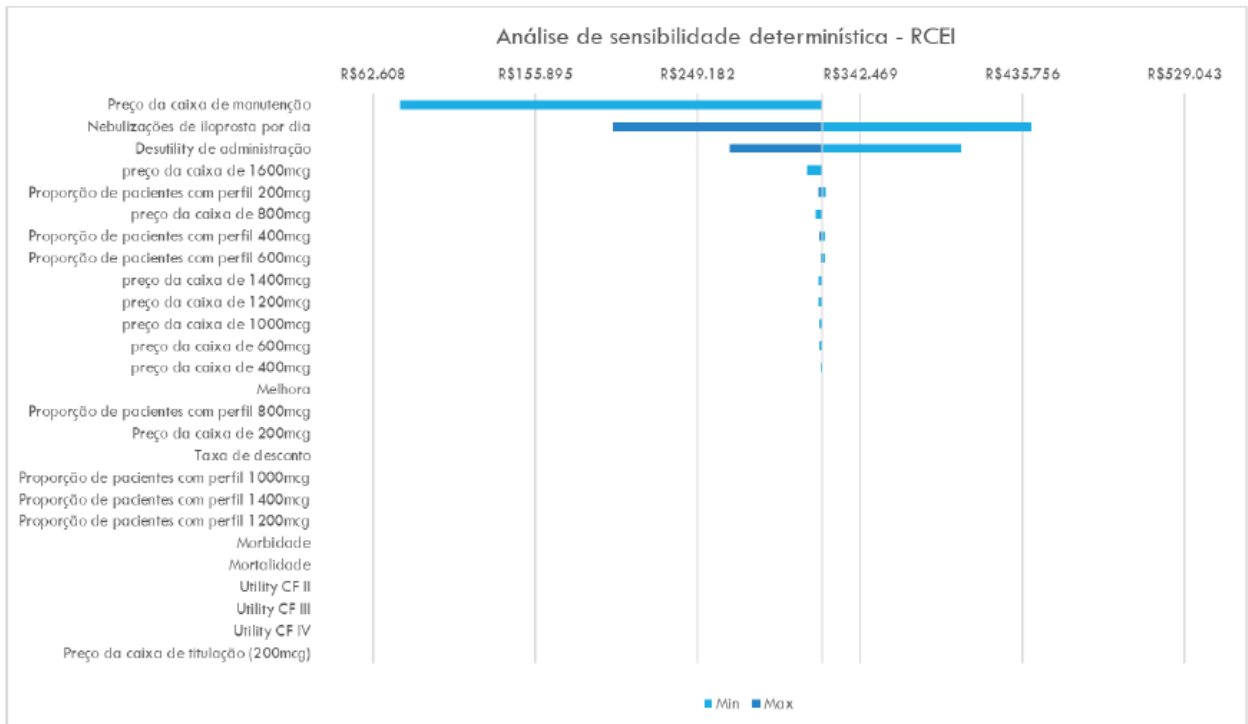
Figura 8: Gráfico de tornado da Análise de Sensibilidade Determinística
