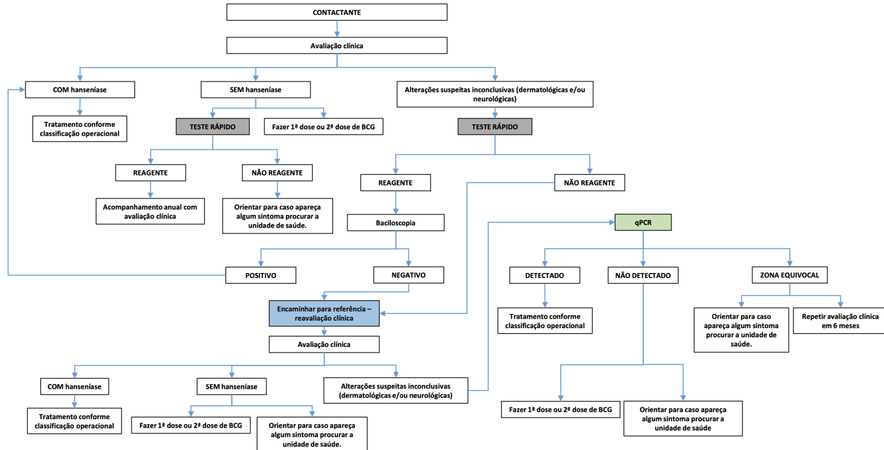
Figura 2. Fluxograma de testes diagnósticos para pacientes suspeitos de hanseníase
