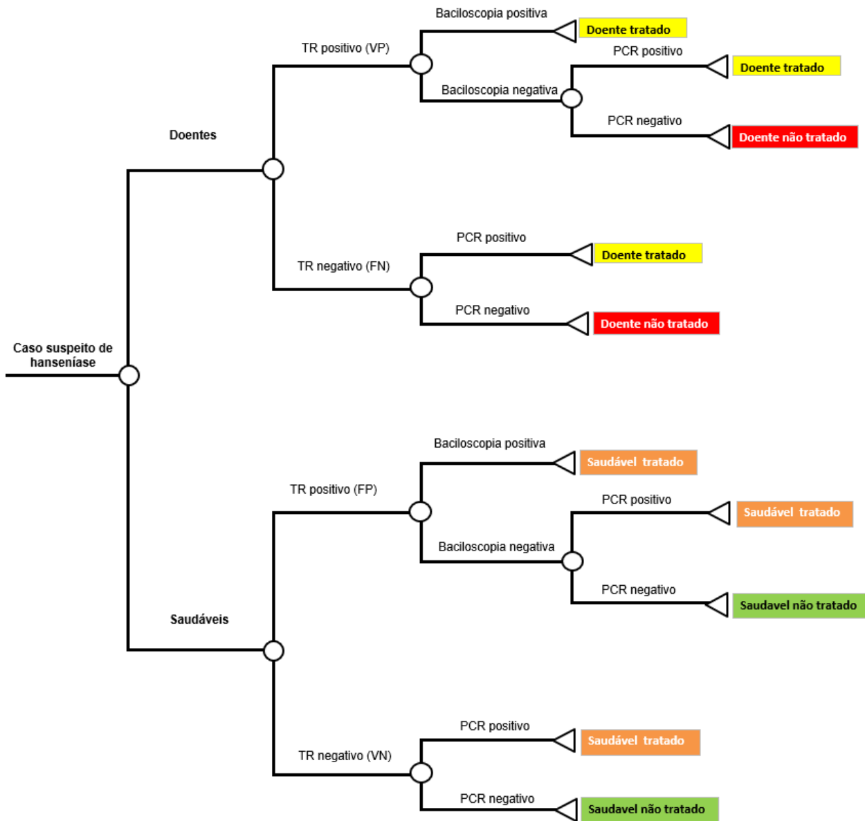
Figura 8. Árvore de decisão para diagnóstico de hanseníase com teste rápido seguido de baciloscopia e PCR
