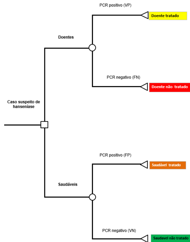
Figura 6. Árvore de decisão para diagnóstico de hanseníase com PCR
