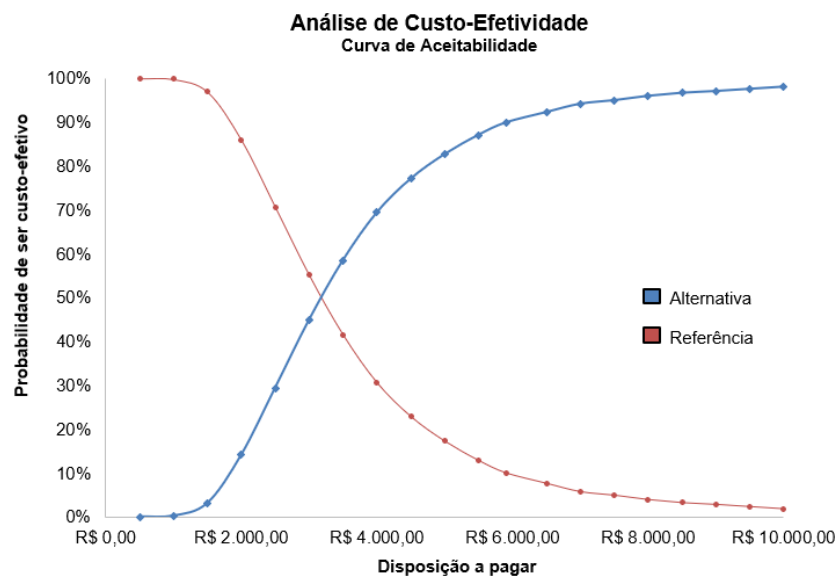
Figura 11. Curva de aceitabilidade do uso sequencial do teste rápido, baciloscopia ou PCR versus o uso isolado de baciloscopia no diagnóstico de hanseníase
