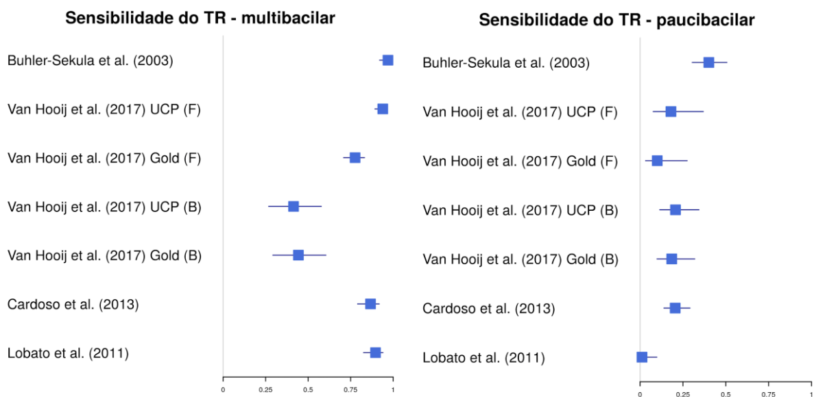
Figura 4. Gráfico de Floresta da sensibilidade do teste rápido para MB e PB
