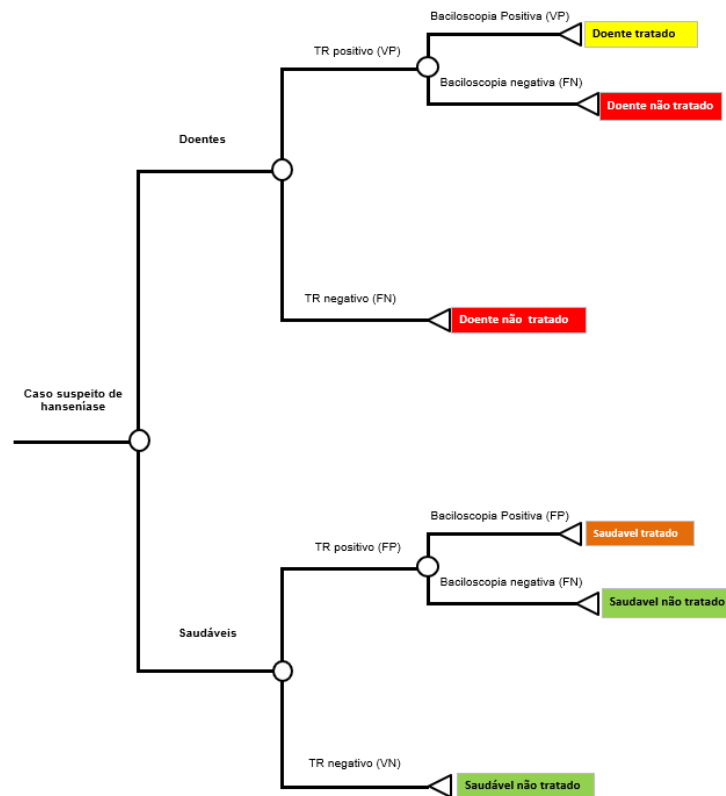
Figura 7. Árvore de decisão para diagnóstico de hanseníase com teste rápido seguido de baciloscopia
