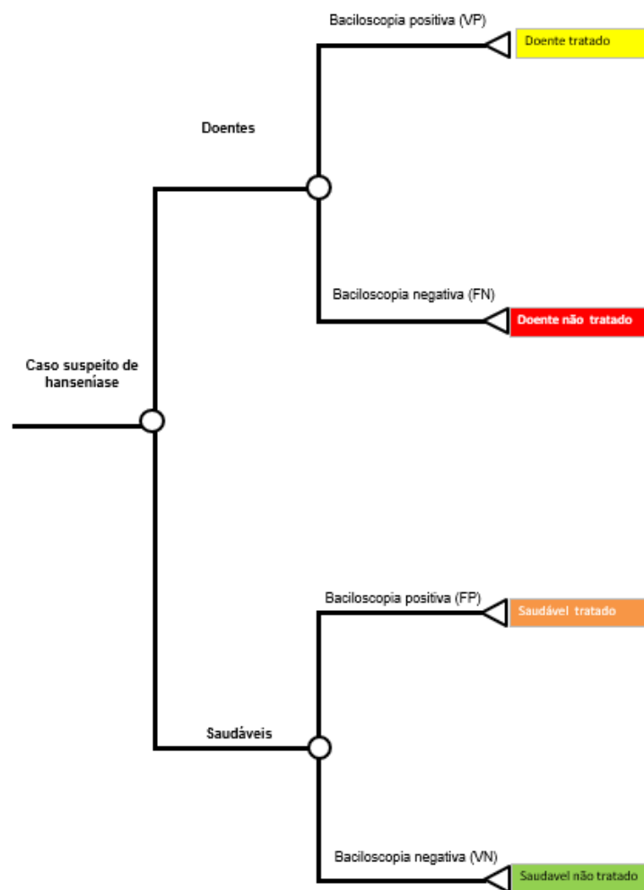
Figura 5. Árvore de decisão para diagnóstico de hanseníase com baciloscopia
