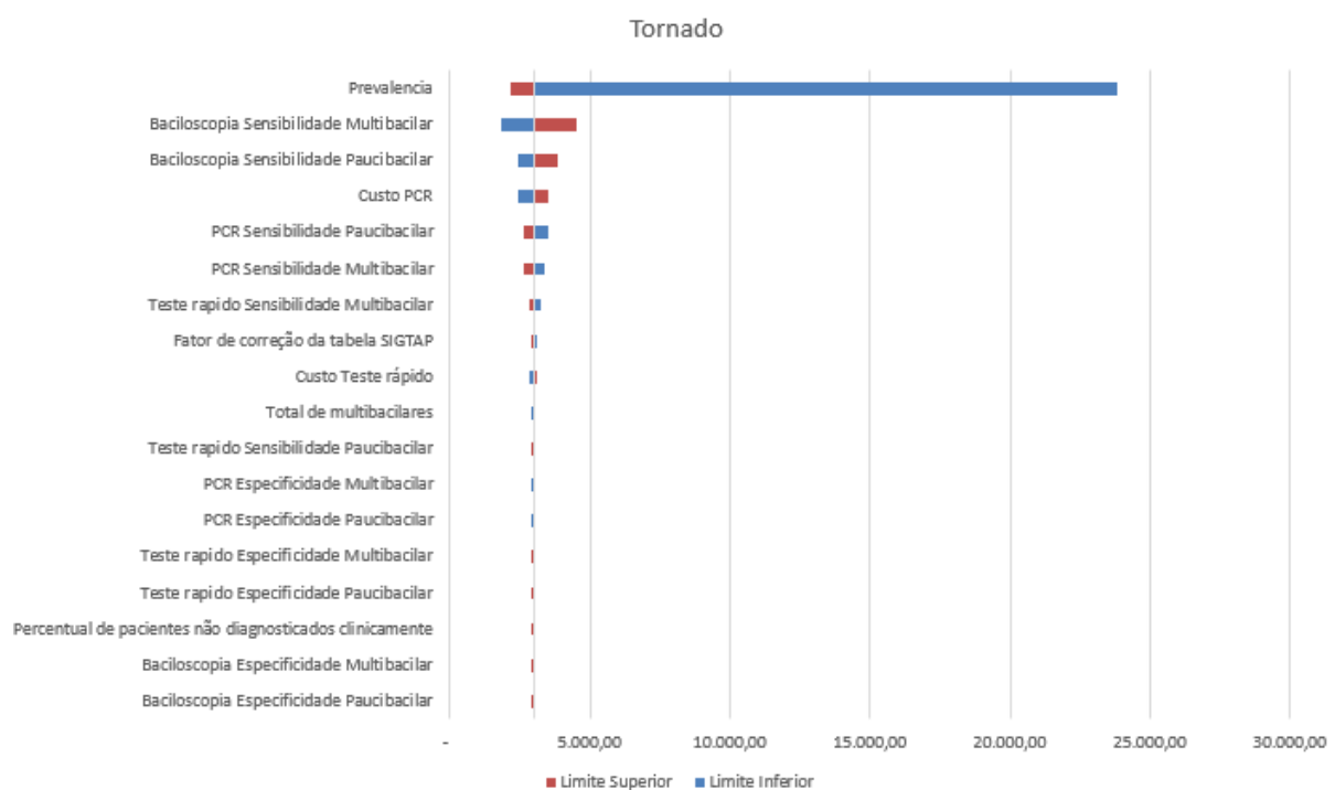
Figura 9. Diagrama de tornado das variáveis utilizadas na análise da RCEI dos testes diagnósticos em hanseníase
