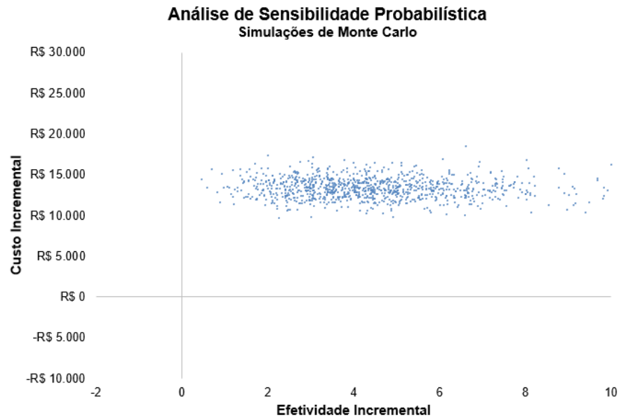
Figura 10. Análise de sensibilidade probabilística das simulações dos testes diagnósticos em hanseníase
