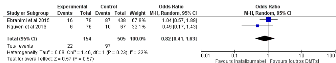
Figura A12 - Forest-plot da meta-análise direta do desfecho de nascimentos prematuros para a comparação natalizumabe vs. outros MMCD Fonte: Centro Colaborador do SUS (CCATES/UFMG), em 2020.
