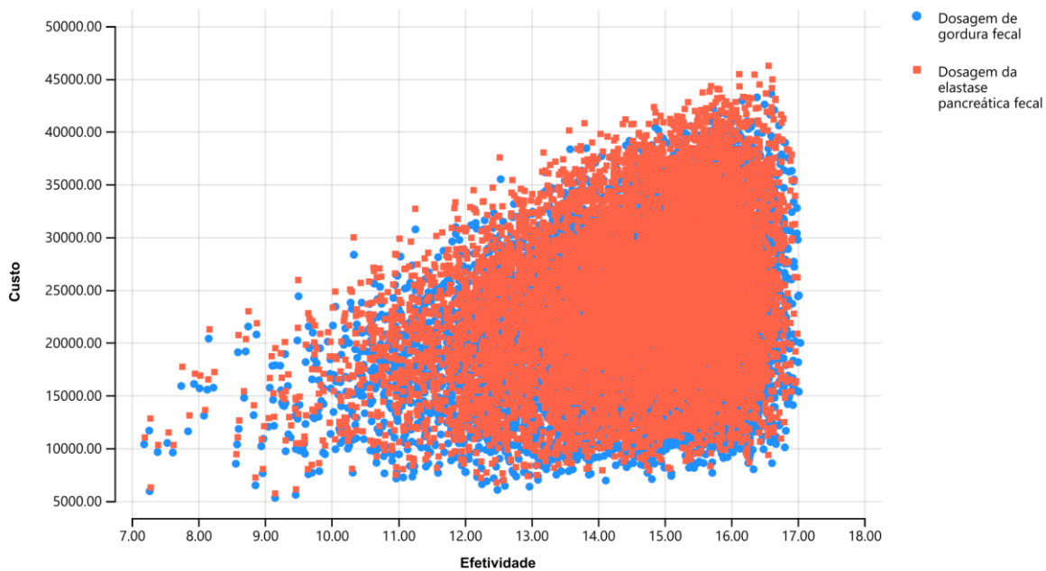
Figura 8. Scatter plot de custo-efetividade.
