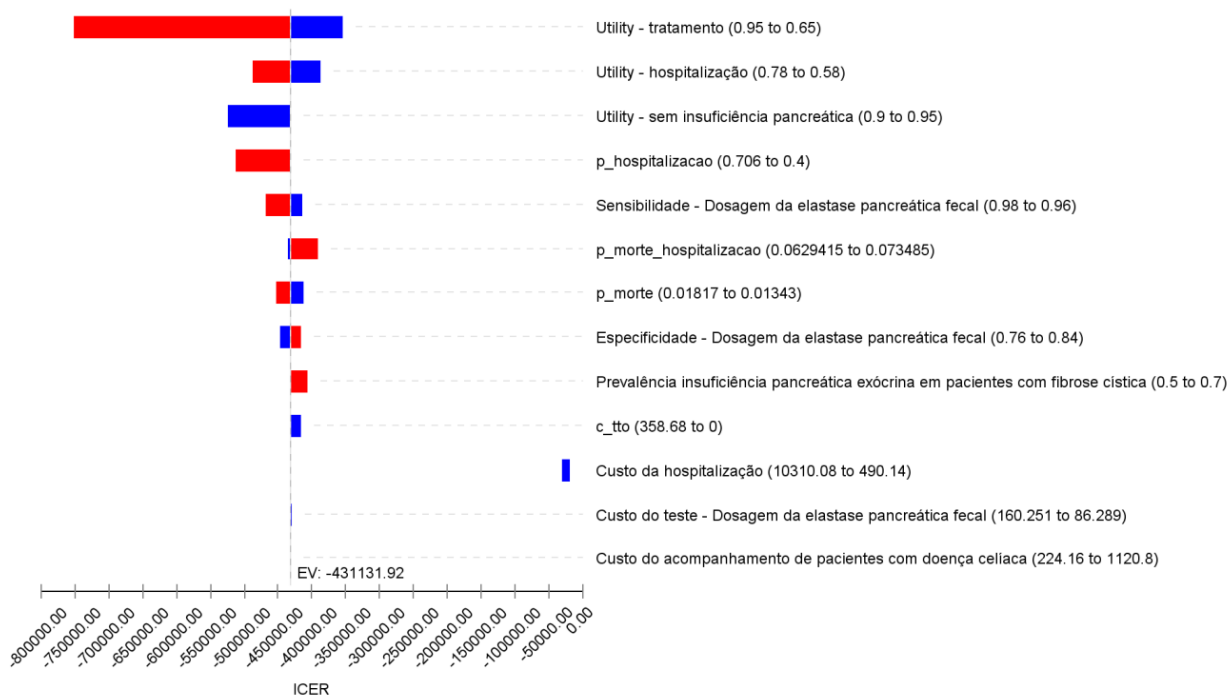
Figura 6. Diagrama de tornado para RCEI.
