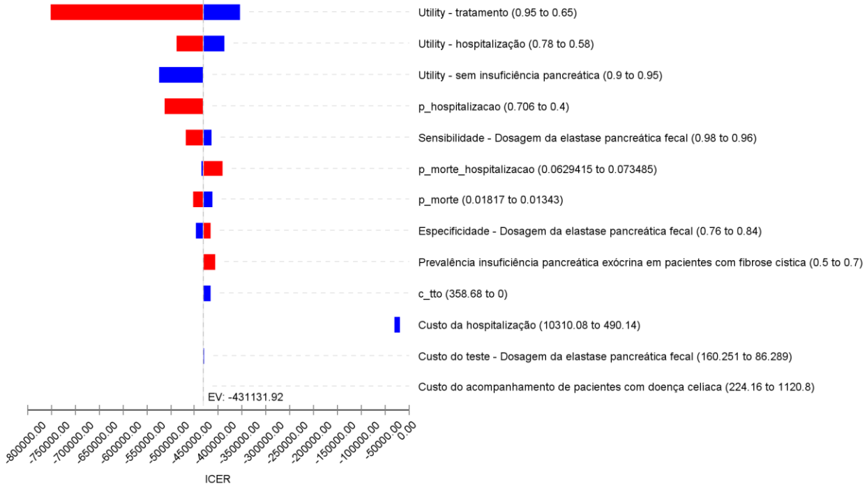
Figura 7. Diagrama de tornado para RCEI.
