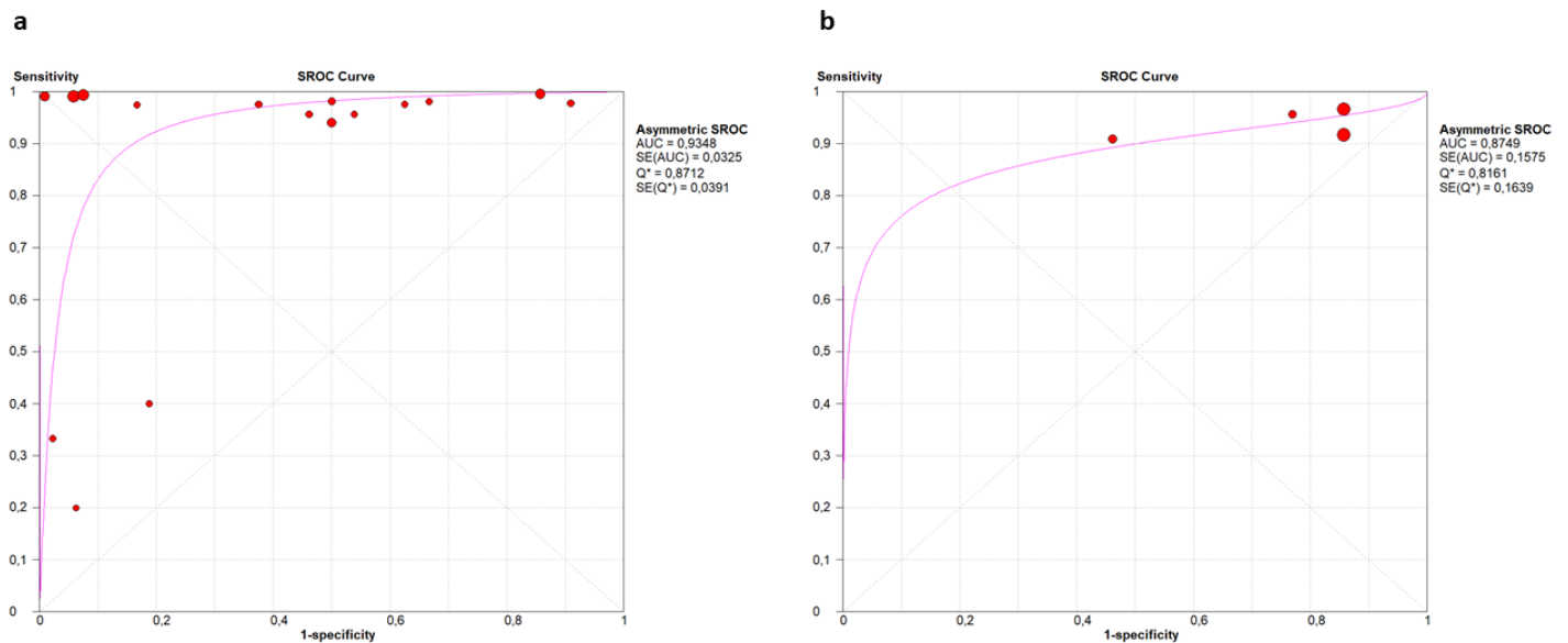
Figura 6. Modelo assimétrico de curva SROC por subgrupo conforme ponto de corte de EL-1 na definição de IPE. a. Estudos que definiram IPE para quantificações \leq 100\mu\text{g} EL-1/g de fezes; b. Estudos que definiram IPE para quantificações < 200\mu\text{g} EL-1/g de fezes.
